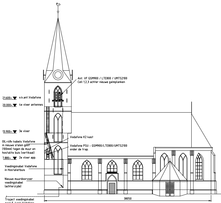
ONTWERP DRAGER ANTENNESYSTEEM STEPHANUSKERK BEILEN
